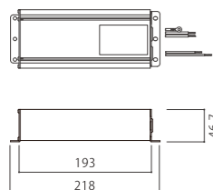
β2-700-130NF 定電流電源 L 700mA
