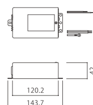
β1-700-65NF 定電流電源 M 700mA
