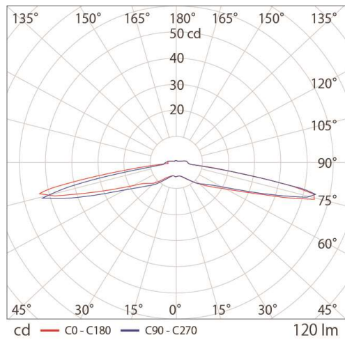
■配光曲線図
