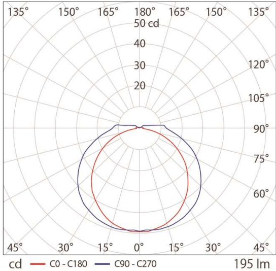
■ 配光曲線図
