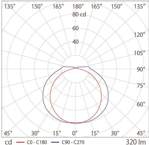
■ 配光曲線図
