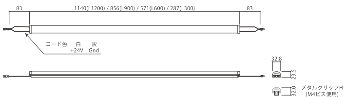
SBX1-△△H30E 電球色 3000K 1940 / 1455 / 970 / 485 lm SBX1-△△H27E 電球色 2700K 1875 / 1410 / 940 / 470 lm
