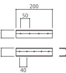
取付ブラケット
