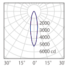
GT6△△-50H 昼白色 5000K 1920 / 1440 / 960lm
