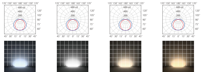
SBX1-△△H65E 昼光色 6500K 2075 / 1555 / 1040 / 520 lm SBX1-△△H50E 昼白色 5000K 2100 / 1575 / 1050 / 525 lm SBX1-△△H40E 白色 4000K 2100 / 1575 / 1050 / 525 lm SBX1-△△H35E 温白色 3500K 2050 / 1540 / 1025 / 515 lm
