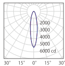
GT6△△-65H 昼光色 6500K 1920 / 1440 / 960lm
