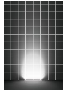
GT6△△-50H 昼白色 5000K 1920 / 1440 / 960lm
