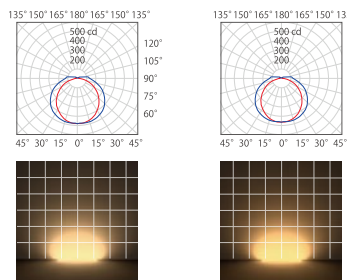
SBX1-△△H30E 電球色 3000K 1940 / 1455 / 970 / 485 lm SBX1-△△H27E 電球色 2700K 1875 / 1410 / 940 / 470 lm
