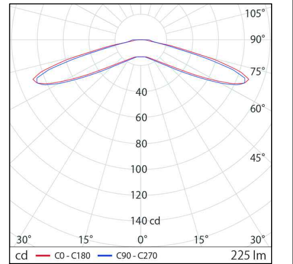
■配光曲線図
