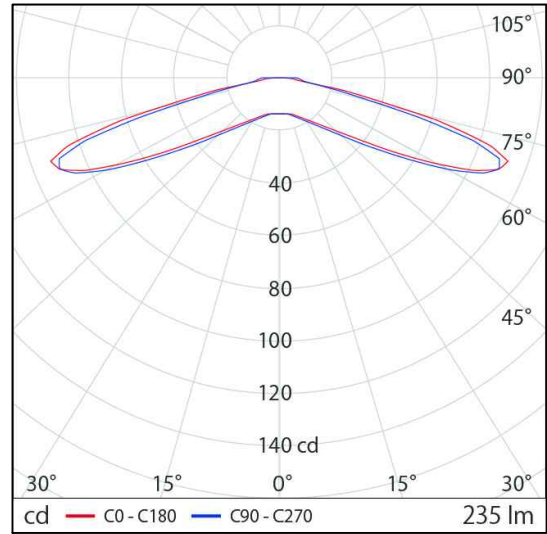
■配光曲線図
