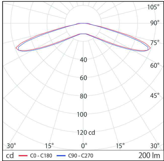
■ 配光曲線図
