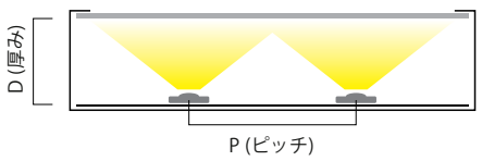
行灯 D : P = 1 : 1.6
