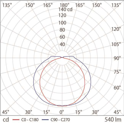
■配光曲線図
