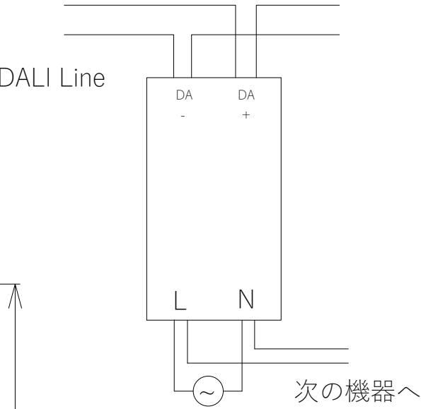
接続図
